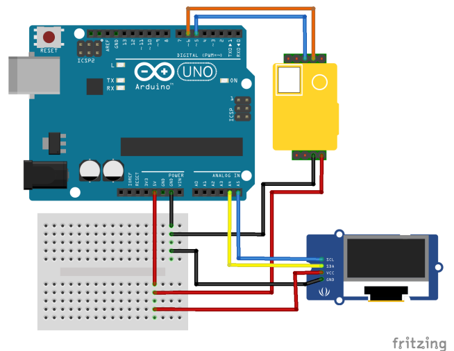
Schaltplan
