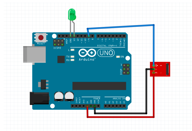
Schaltplan
